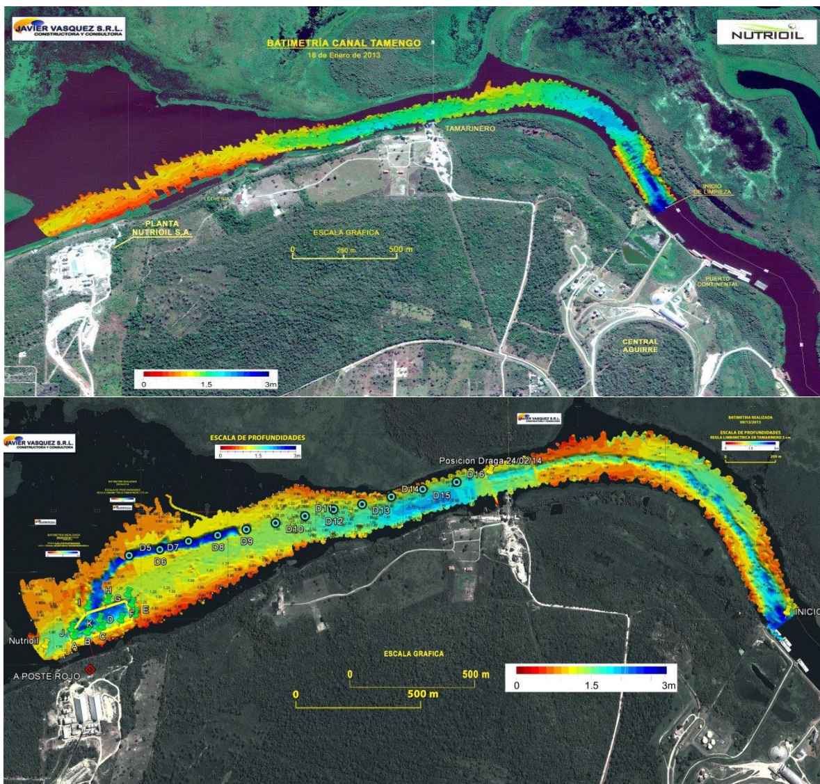
Gráfico No. 2 Fotografía Satelital – Estudios de Batimetría a Enero de 2013 y a Marzo de 2014
