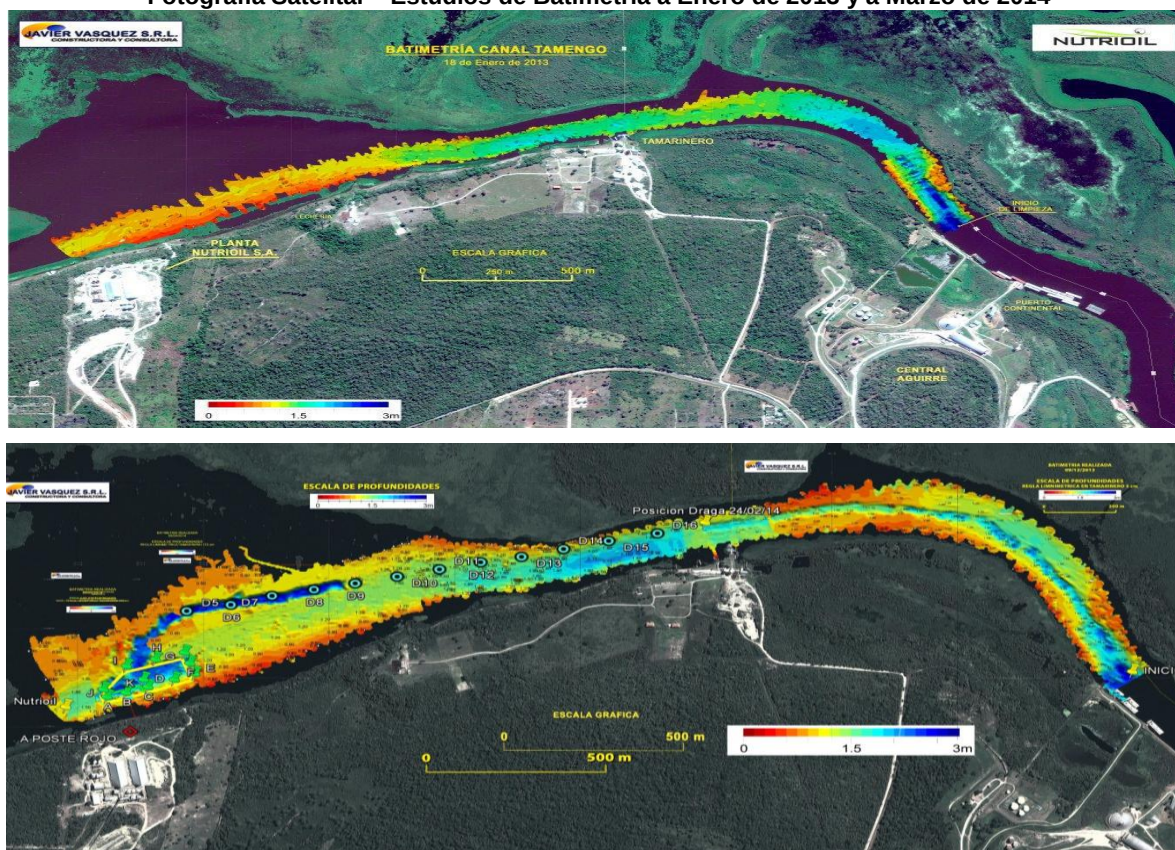
Fotografía Satelital – Estudios de Batimetría a Enero de 2013 y a Marzo de 2014
